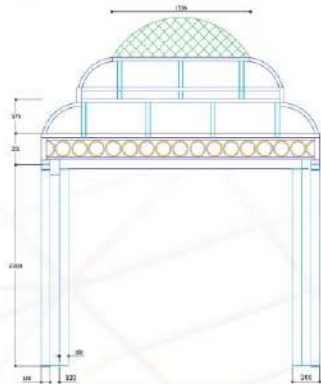
LEFT ELEV. Scale: 1/50
