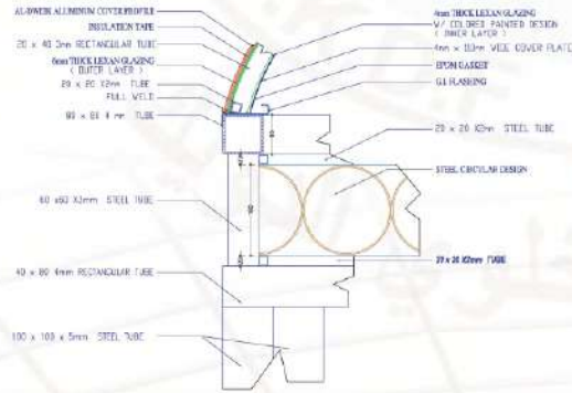
SEC. DET. "SI" Scale: 1/5
